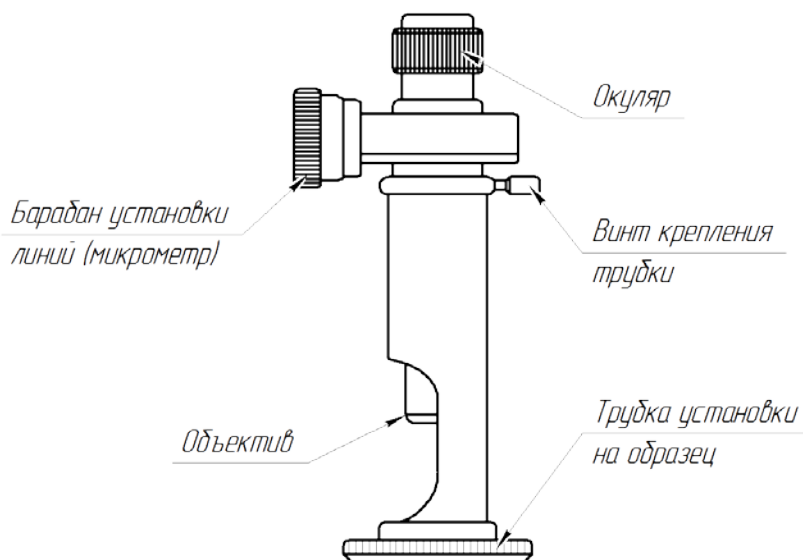
Рисунок 2.3 – Измерительный микроскоп
